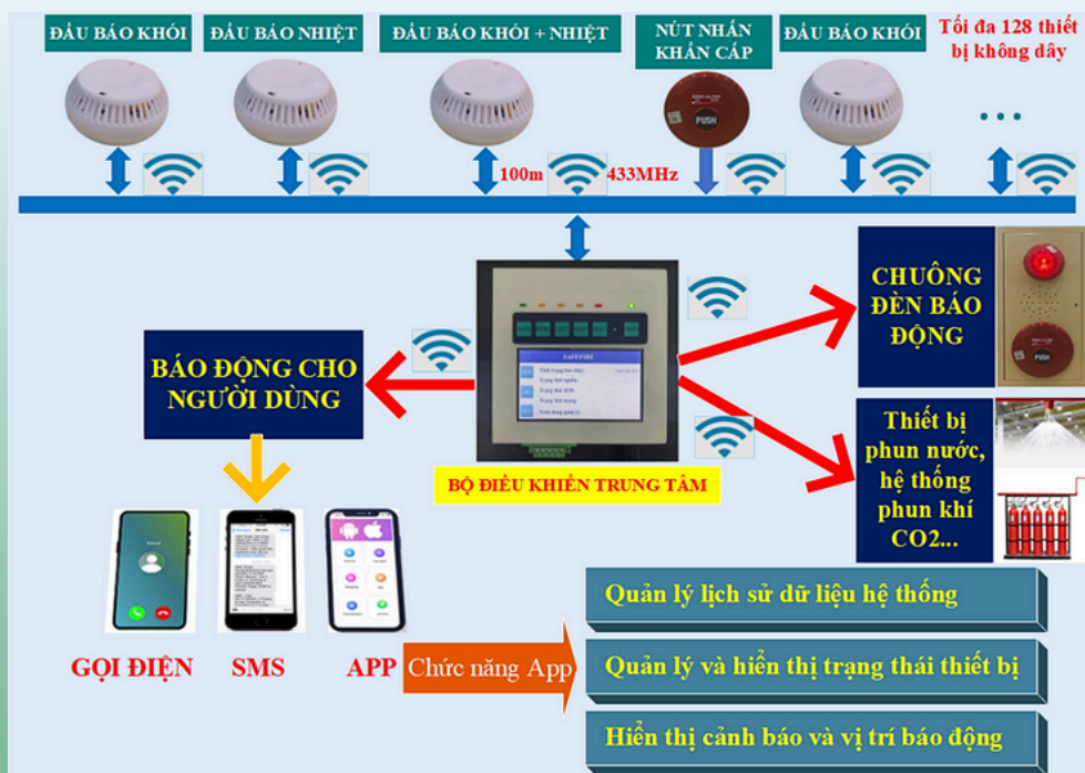
Hệ thống báo cháy không dây do AIOT phát triển
